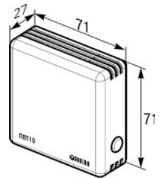
Рисунок 3.1 – Габаритные размеры
